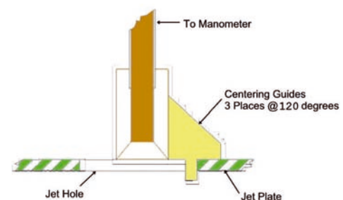
Fig. 3 Probe
