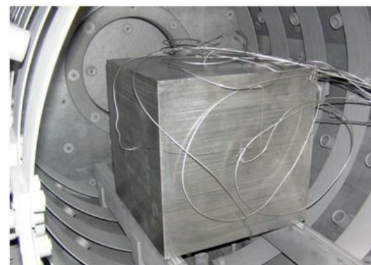
Rys. 3. Próba szybkości chłodzenia wg NADCA na referencyjnym bloku stalowym o wymiarach 400/400/400 mm.
