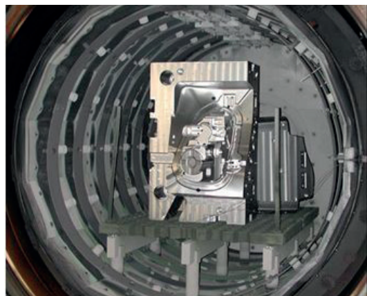
Rys.4. Matryca w komorze pieca próżniowego po kompleksowej obróbce cieplnej.
