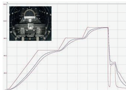
Rys. 2. Przebieg procesu austenizacji i hartowania z przystankiem izotermicznym, z monitoringiem temperatury pieca oraz powierzchni i rdzenia matrycy.
