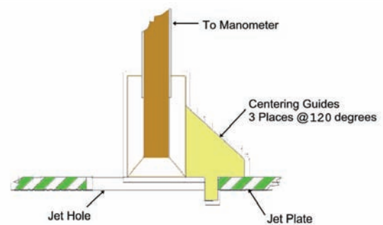
Fig. 3 Probe
